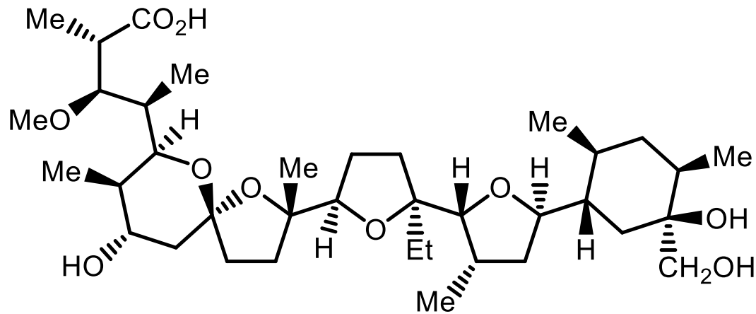
Monensin
